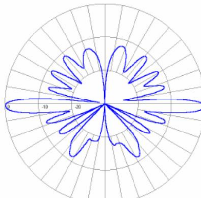
Elevation
